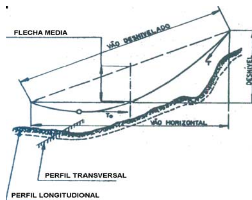
Figura 1: Catenária
